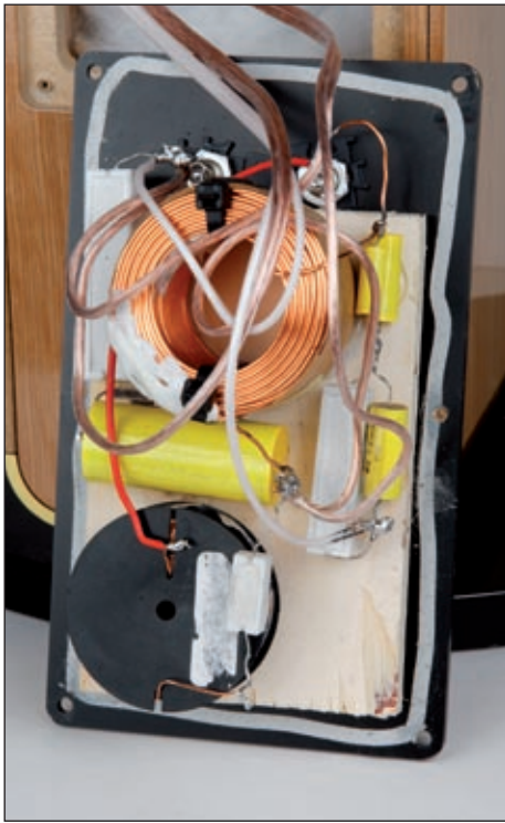
Yhdeksästä elementistä huolimatta Graphican jakosuodin on pelkistetty, koska se jakaa alueen vain kahteen kaistaan.
